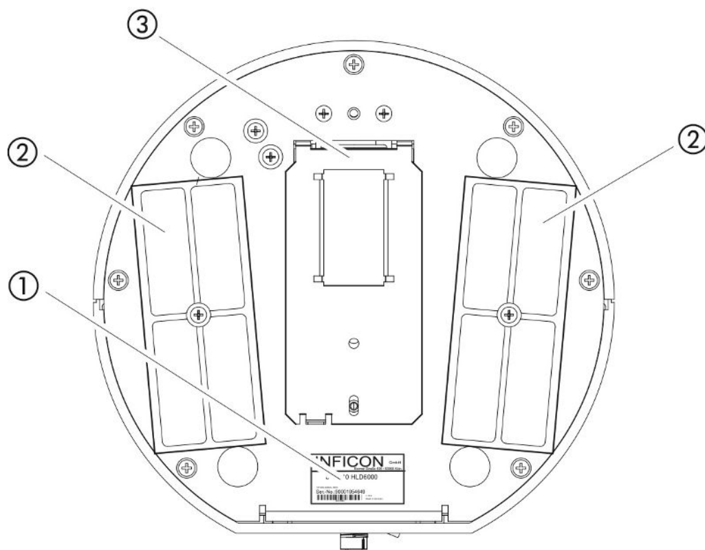
図 3: ボトムビュー
