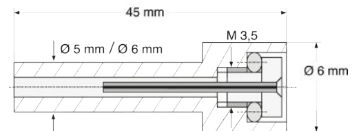
Kalibrierleck mit Einschraubhülse
