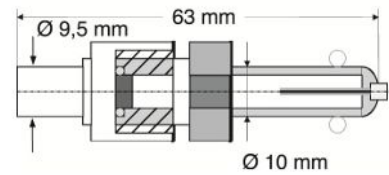
Kalibrierleck mit zylindrischem Gehäuse und VCO-Anschluss
