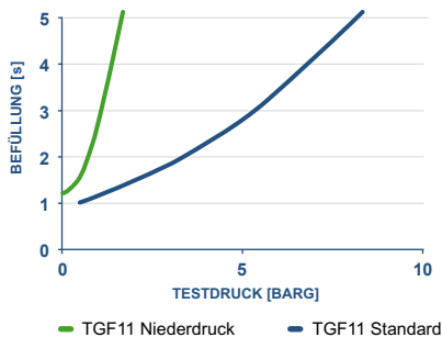
Befüllung (T90) eines 5-Liter-Objekts
