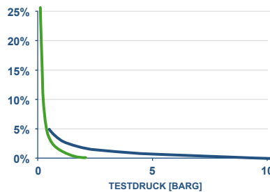
Maximale Drucküberschreitung
